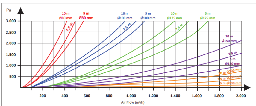
Painehäviökäyrät:
